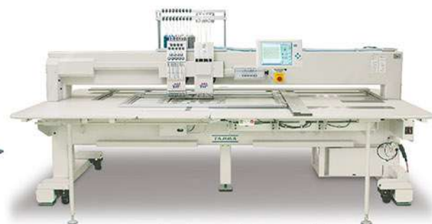
PAX 冲孔, 缝纫和刺绣 多功能一体机
