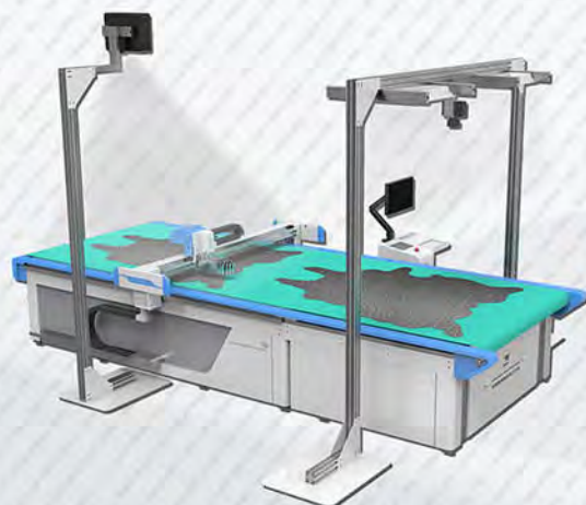
锦德摄像+投影真皮裁切机器人
